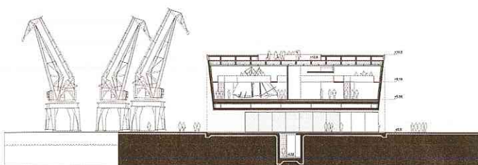
PRZEKRÓJ M. 1:1.000
