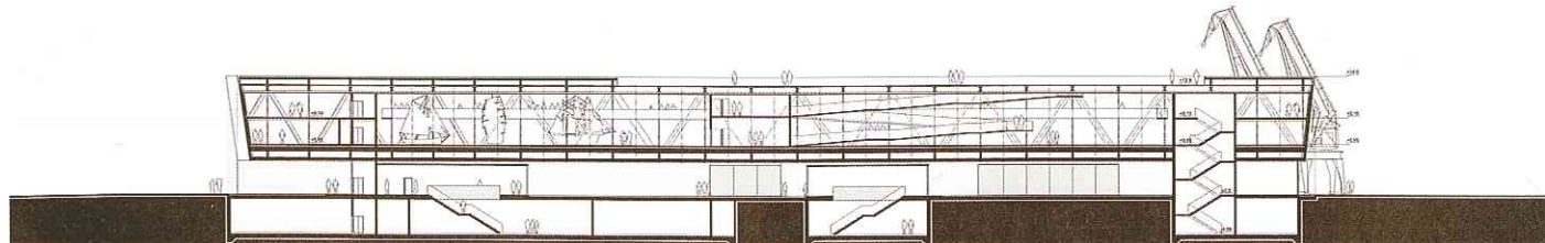
PRZEKRÓJ A-A M. 1:1.000
